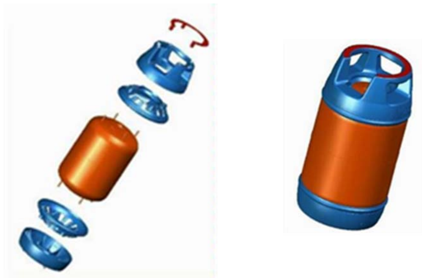
Фиг. 8 – Изделие «Баллон для газа и его части».
